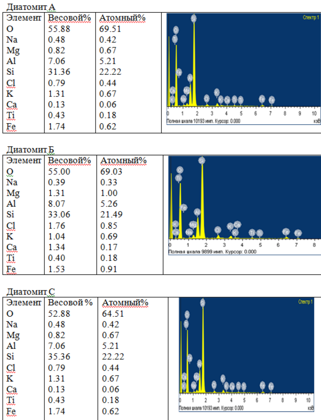
Рисунок 2 – Результаты растрового электронного микроскопирования
